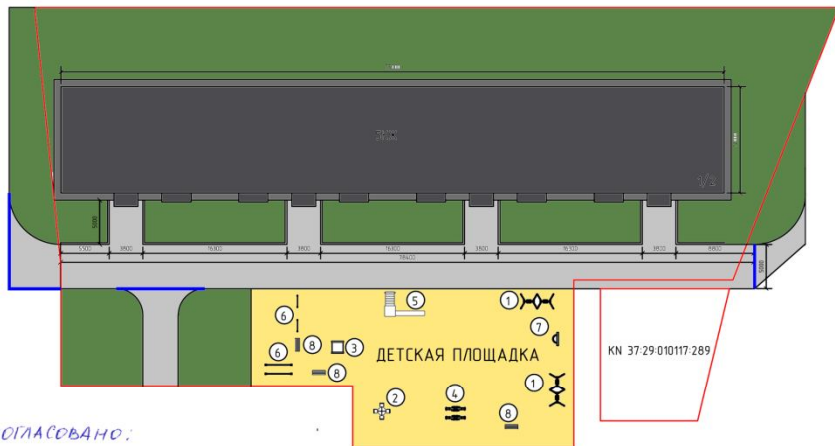
План благоустройства дворовой территории М 1:500
